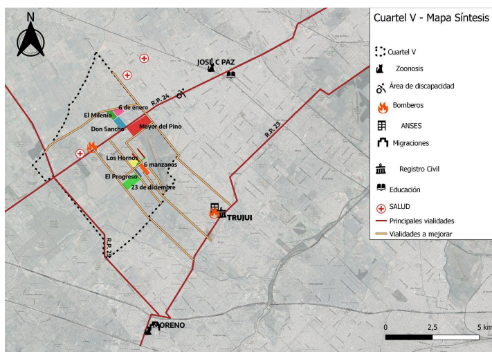
Figura 3. Mapa síntesis
